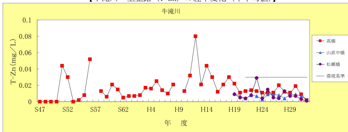
【牛滝川 全亜鉛（T-Zn）の経年変化（年平均値）】
