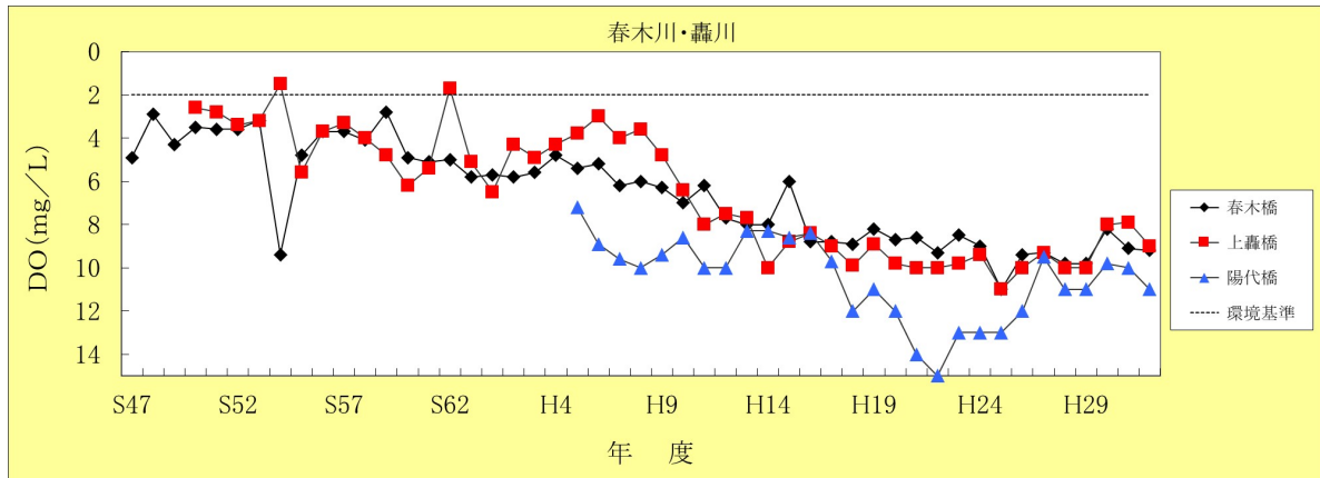
【春木川、轟川 溶存酸素量 (D0) の経年変化 (年平均値)】
